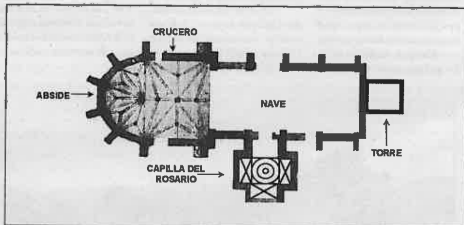
PLANTA ACTUAL DE LA IGLESIA PARROQUIAL
