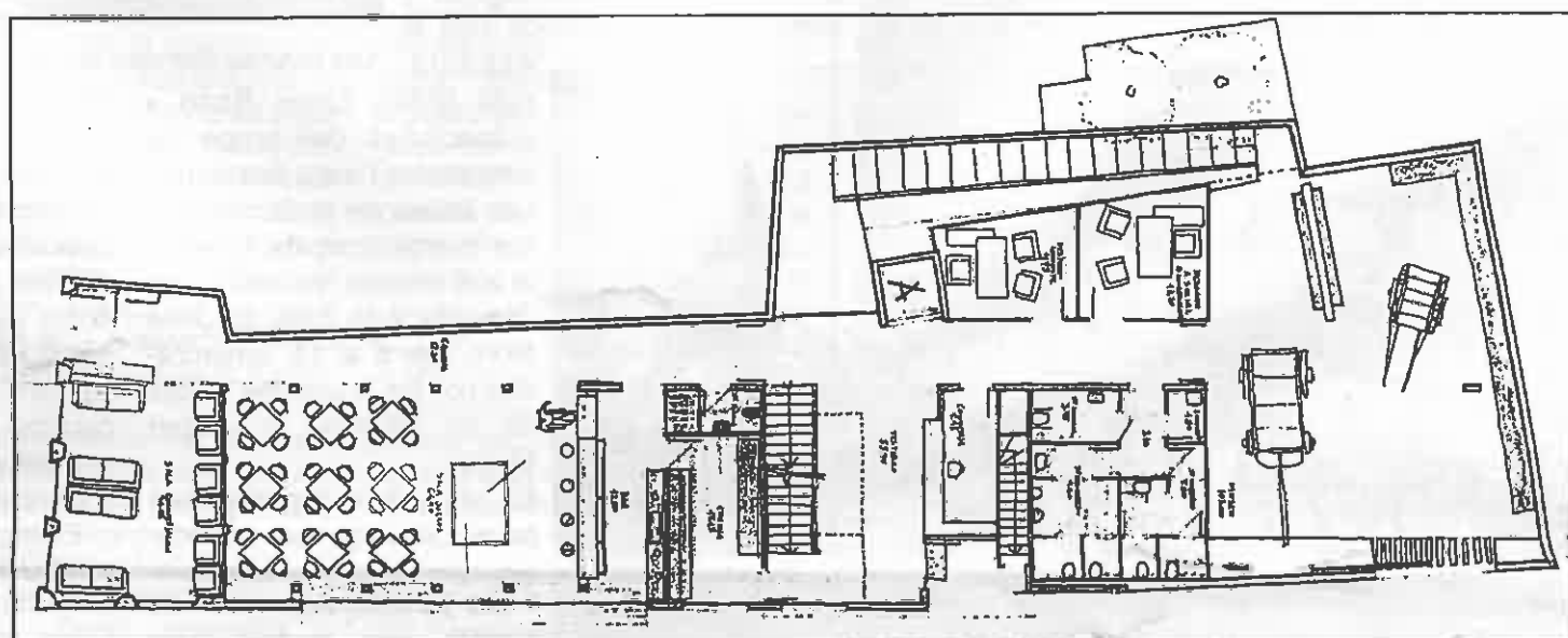
PLANTA BAJA
